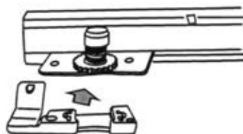
Правая направляющая
